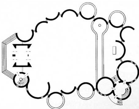
Ryc. 227. Kościół Najświętszej Marii Panny Matki Kościoła w Poznaniu-Świerczewie – rzut przyziemia
