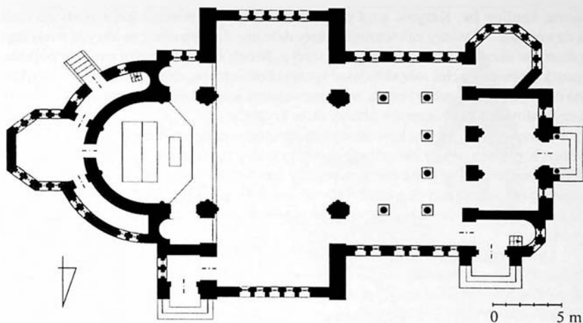
Ryc. 18. Wiry, kościół św. Floriana (1900 r.) – rzut przyziemia
