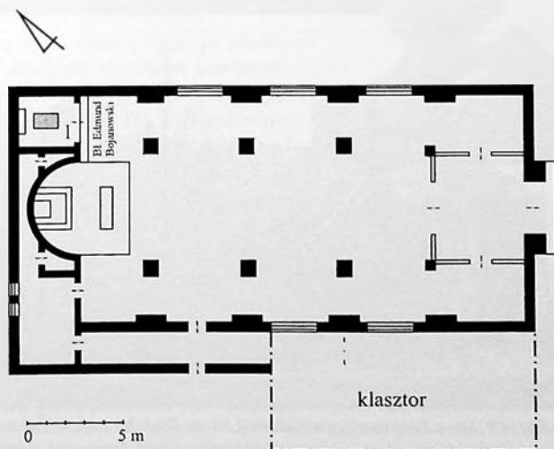
Ryc. 46. Żabikowo, kaplica Najśw. Serca Jezusa – rzut przyziemia (1 – grób bł. Edmunda Bojanowskiego)
