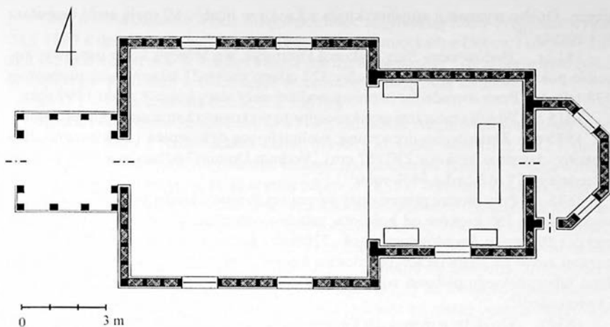
Ryc. 8. Stary kościół w Wirach pod koniec XIX w. (rzut przyziemia)
