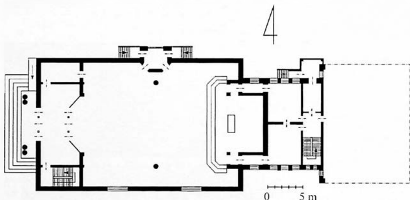
Ryc. 195. Kościół (II) św. Maksymiliana Marii Kolbe w Luboniu-Lasku, rzut przyziemia (w budowie od 2001 r.)
