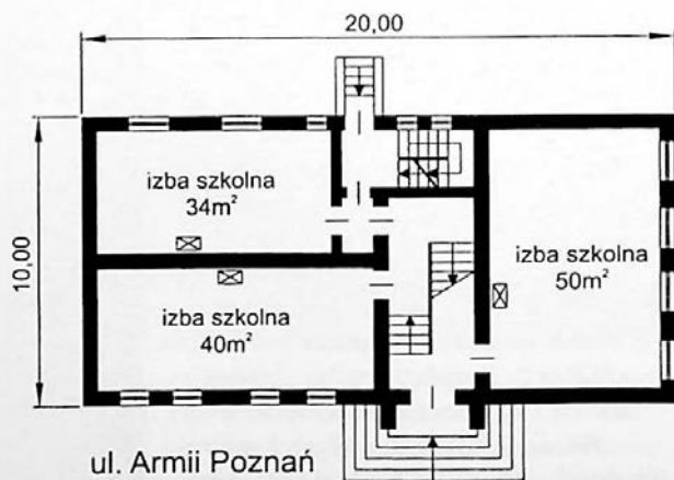
Ryc. 300. SP nr 3 – rzut parteru (1905 r.)
