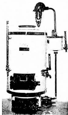
Ryc. 509. Samowar typ „Gigant” (model z 1961 r.; opracowany przez ZDZ) do wagonów osobowych
