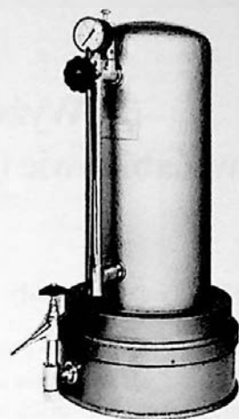
Ryc. 515. Saturator bufetowy typ SP1/A do wytwarzania wody sodowej z manometrami zagazowania wody CO 2 o wydajności 140 l/h
