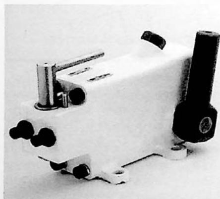
Ryc. 512. Pompy hydrauliczne do podnoszenia kabiny samochodów średniej i dużej ładowności (typ: PTR 3,5 i PTR 5,3)
