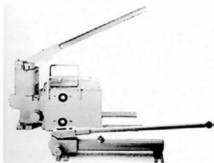
Ryc. 510. Pompy hydrauliczne do napędu siłowników (typ PTR 2,3 i dwustopniowa typ PTR 118,5/5)
