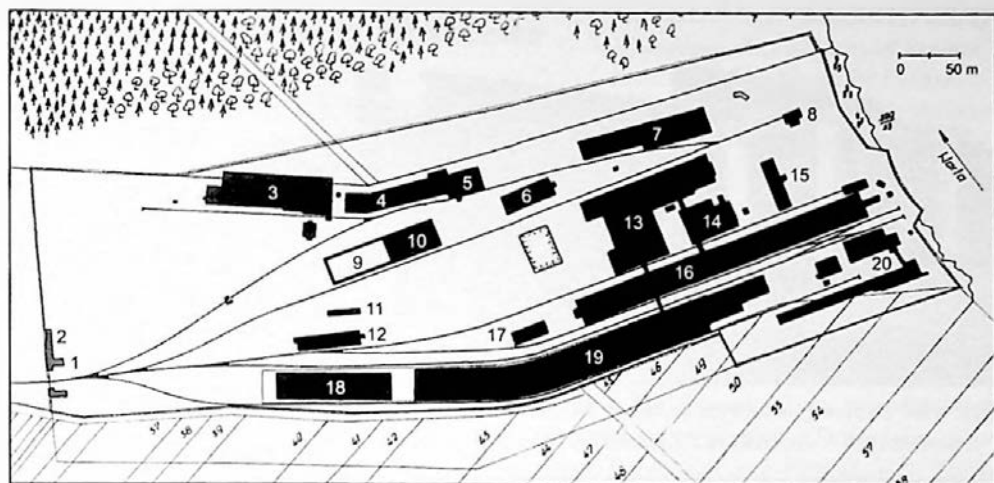
Ryc. 494. Zakłady Chemiczne im. R. Maya w Luboniu – lokalizacja szkoły (1948 r.): 1 – portiernia, 2 – straż pożarna, 3 – wytwórnia kwasu siarkowego II, 4 – skład pirytu, 5 – wytwórnia kwasu siarkowego I, 6 – zbiorniki kwasu siarkowego, 7 – wytwórnia soli fosforowej, 8 – parowozownia, 9 – SZKOŁA, 10 – garaże, 11 – budynek gospodarczy, 12 – świetlica, 13 – fabryka superfosfatu, 14 – kotłownia, 15 – warsztat naprawczy, 16 – młyny i skład fosforytów, 17 – budynek administracyjny, 18 – stołówka-laboratorium, 19 – skład superfosfatu, 20 – wytwórnia kleju
