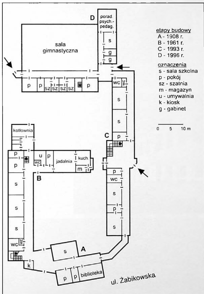
Ryc. 246. SP nr 2 – rzut parteru (2000 r.)
