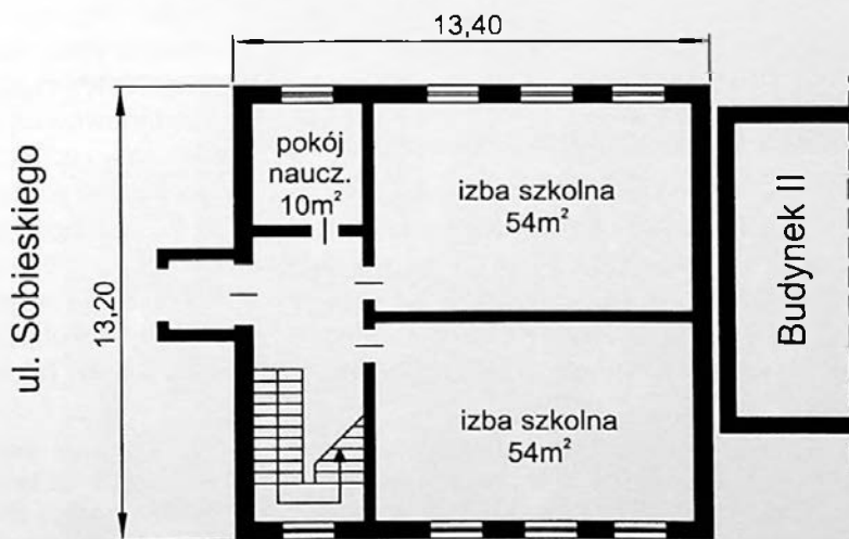
Ryc. 109. SP nr 4 – budynek III, rzut parteru (1931–2001)
