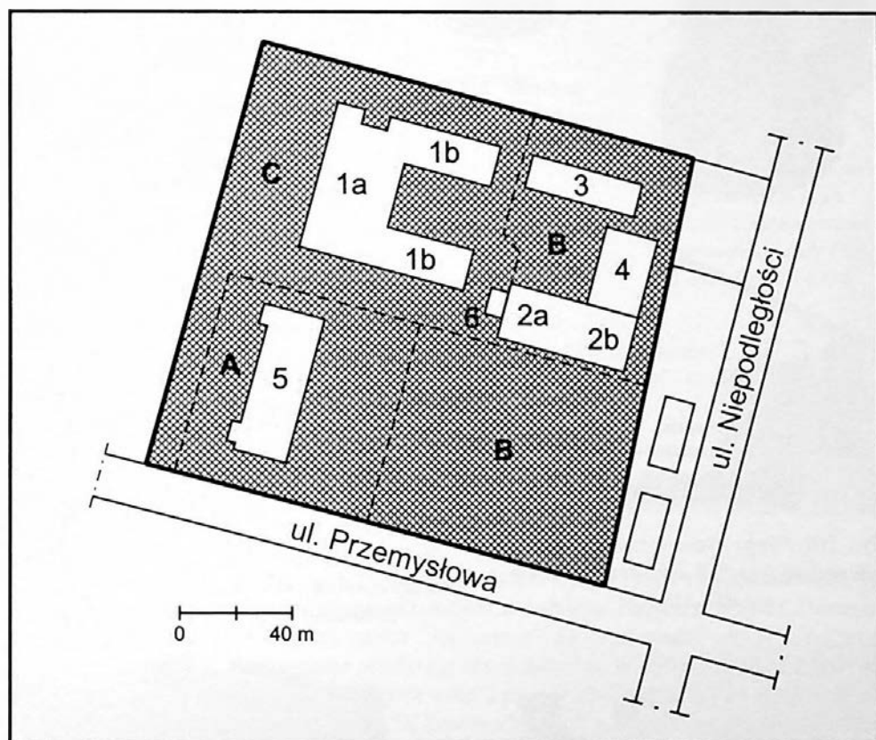
Ryc. 507. Warsztat Szkoleniowo-Produkcyjny w Luboniu ul. Przemysłowa 2: 1a – biura i zaplecze socjalne, 1b – warsztat ślusarski, blacharski i mechaniczny, 2a – magazyn, 2b – baza transportowa z placem na 20 samochodów ciężarowych, 3 – krawalnia i spawalnia, 4 – rozbieralnia akumulatorów, 5 – warsztat elektrotechniczny i warsztat sekcji samochodowej, 6 – trafostacja. Podział terenu po likwidacji szkoły: A – firma „Pozbud”, B – firma „Niedźwiedź Lock”, C – firma „Multichem”
