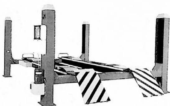
Ryc. 511. Samochodowy podnośnik diagno- styczny czterokolumnowy dla pojazdów o masie całkowitej do 3,5 t (typ. PSD-3,5)
