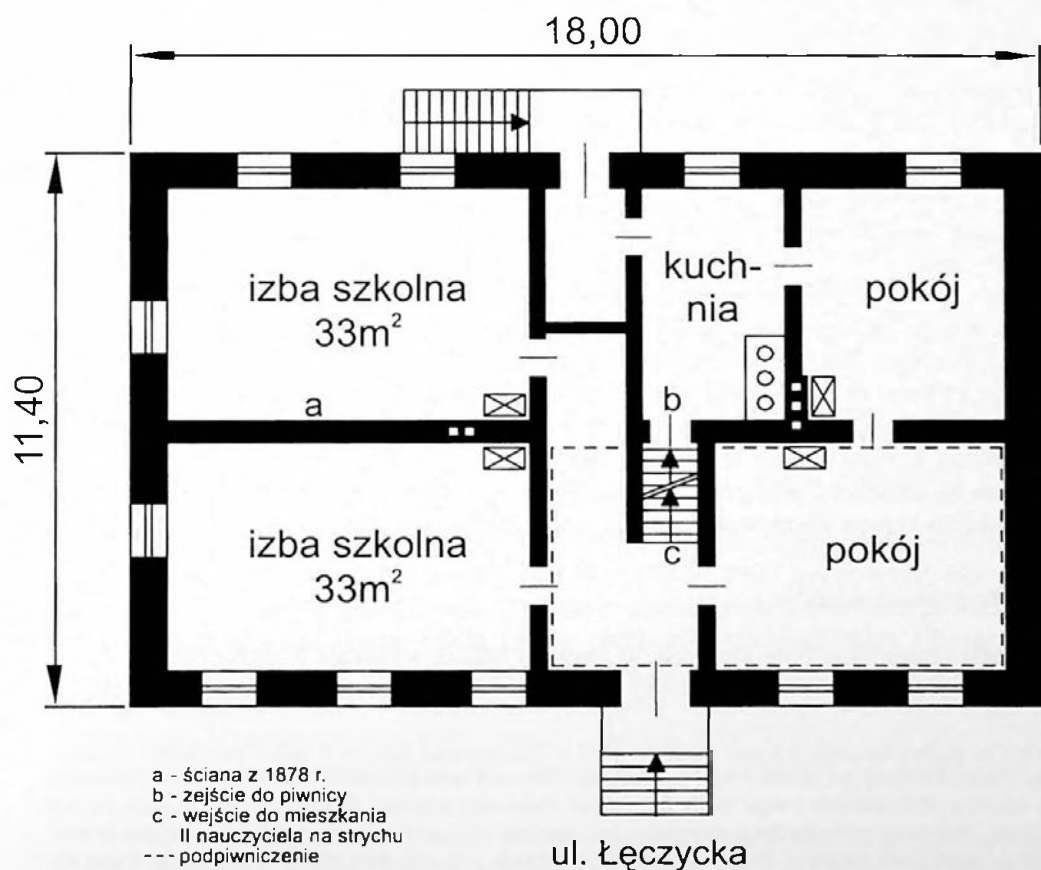
Ryc. 71. Szkoła Podstawowa w Wirach – budynek III, rzut parteru (1847–1912)
