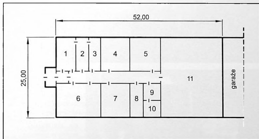
Ryc. 495. Budynek szkolny w Zakładach Chemicznych im. R. Maya w Luboniu: 1 – szatnie, 2 – ustępy, 3 – natryski, 4, 5, 6, 7 – sale szkolne, 8 – kotłownia, 9 – sekretariat, 10 – kierownik, 11 – warsztat szkolny (1948 r.)
