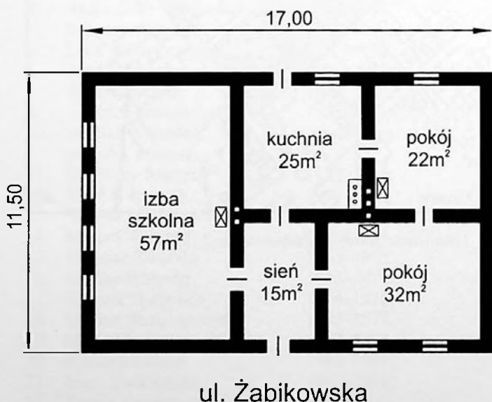
Ryc. 177. SP nr 2 – budynek I, rzut parteru (1845–1906)
