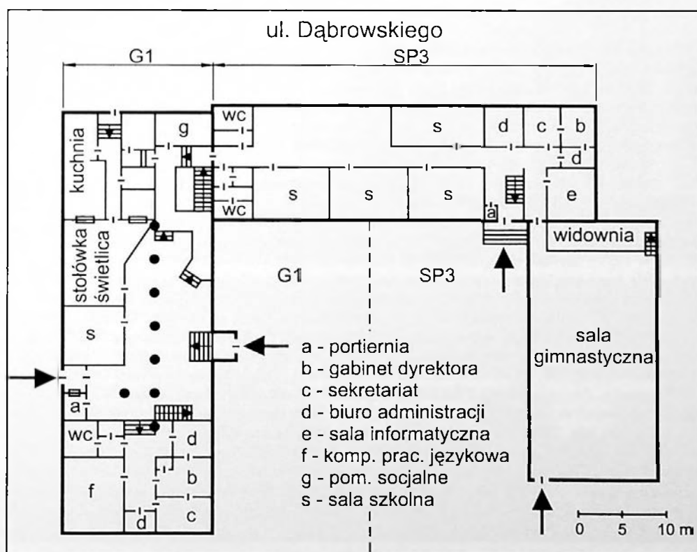
Ryc. 364. Szkoła Podstawowa nr 3 oraz Gimnazjum nr 1 – rzut parteru (2000 r.)
